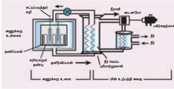
படம் 6.7 அணுக்கரு உலை
