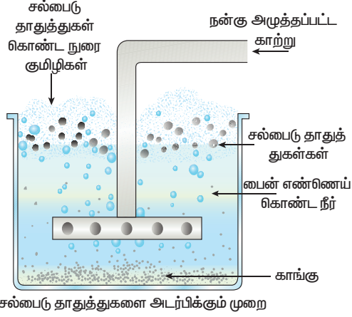
சல்பைடு தாதுத்துகளை அடர்த்திக்கும் முறை
