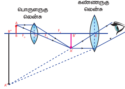
படம் 2.19 கூட்டு நுண்ணோக்கியில் பிம்பம் உருவாதல்
