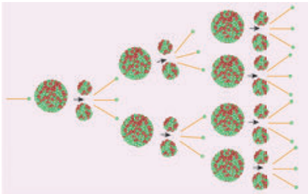
படம் 6.3 கட்டுப்பாடற்ற தொடர்வினை
