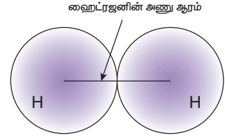
படம் 8.3 ஹைட்ரஜனின் அணு ஆரம்
