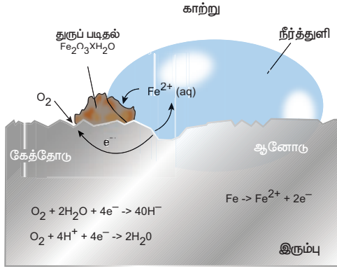
படம் 8.11 துருப்பிடித்தல்
