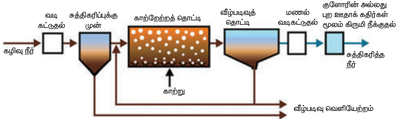
படம் 22.4 கழிவு நீர் சுத்திகரிப்பின் பல்வேறு நிலைகள்
