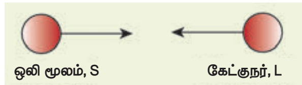
படம் 5.7 ஒலி மூலமும் கேட்குநரும் ஒருவரையொருவர் நோக்கி நகர்தல்
