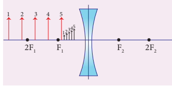
படம் 2.14 குழிலென்சு-பொருளின் தொலைவைப் பொறுத்து பிம்பத்தின் அளவும், தொலைவும் மாறுபடுதல்.
