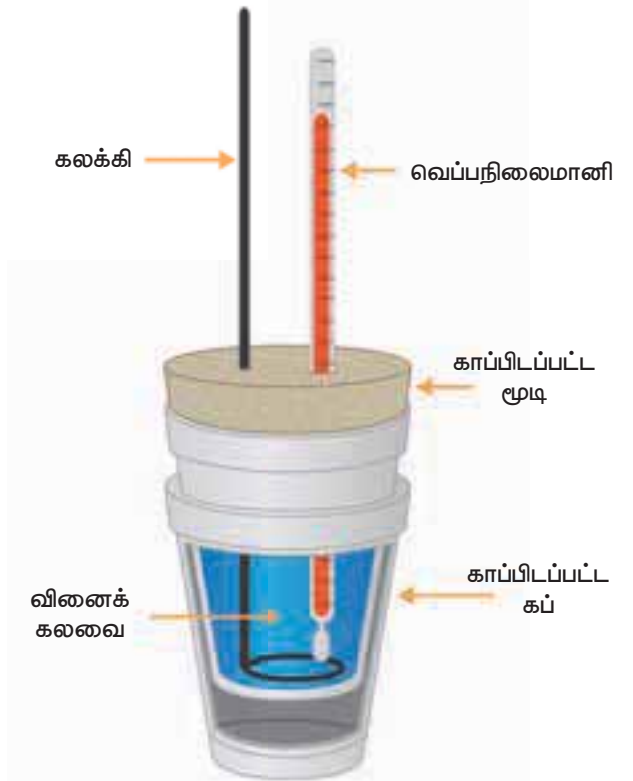
படம்: 7.7 காபி கப் கலோரிமீட்டர்
