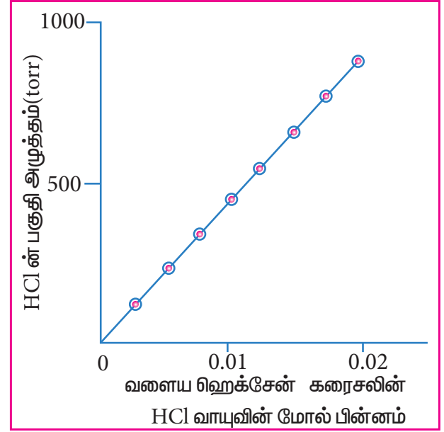
படம் 9.3 293K ல் வளையஹெக்சேனில் கரைந்துள்ள HCl வாயுவின் கரைதிறன்
