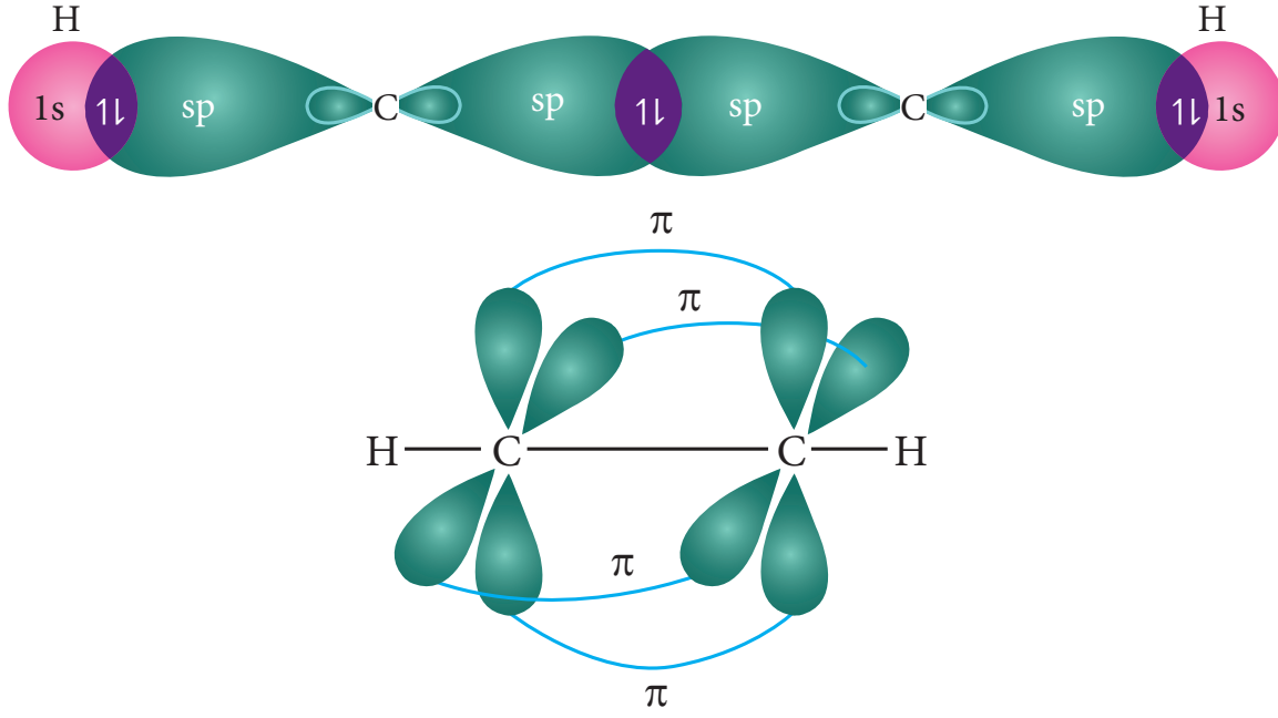
படம் 10.28 அசிட்டிலீனில் sp இனக்கலப்பு
