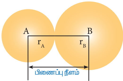
படம் 10.13 A - B சகப்பிணைப்பு மூலக்கூறின் பிணைப்பு நீளம்
