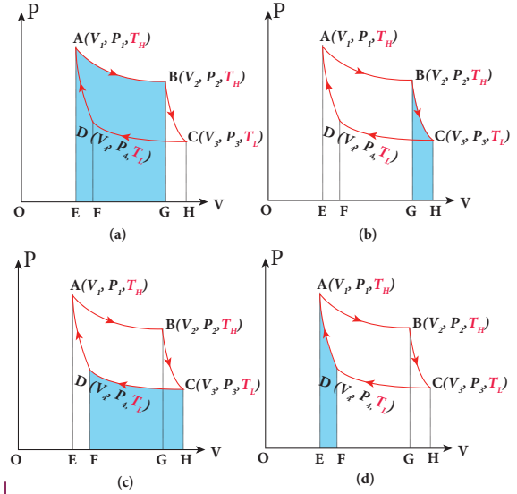
படம் 8.46 கார்னோ சுற்றில் செய்யப்பட்ட வேலை
