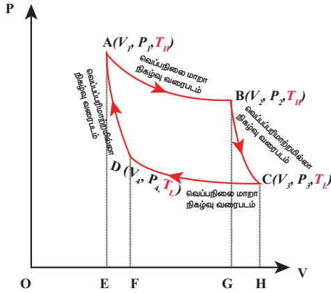
படம் 8.45 கார்னோ சுற்றுக்கான PV வரைபடம்
