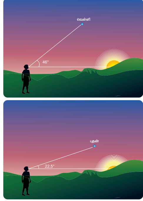
படம் 6.28 அடிவானத்திலிருந்து வெள்ளியின் ஏற்றக் கோணம்
