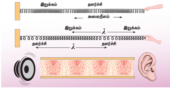
படம் 11.12 நெட்டலையின் அலைநீளம்
