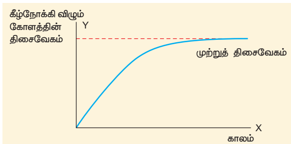
படம் 7.18 திசைவேகம் – காலம் வரைபடம்
