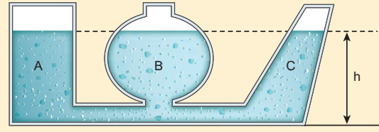
படம் 7.11 நீர்மநிலையியல் முரண்பாடு விளக்கம்
