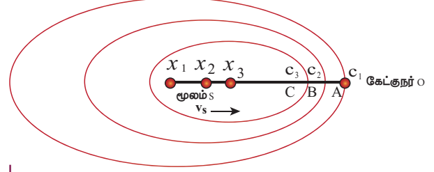
படம் 11.46 மூலம் (S) ஒய்வில் உள்ள கேட்பவர் (O) வலது புறம் ஒரு திசைவேகத்தில் நெருங்கும்போது v_s
