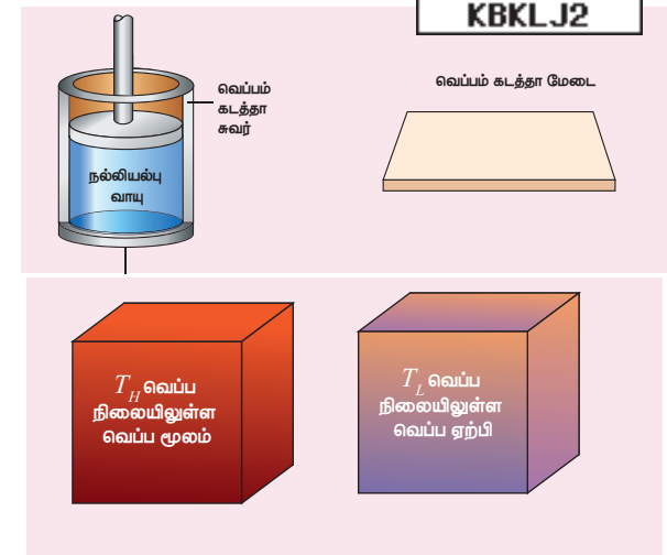
படம் 8.44 கார்னோ இயந்திரம்
