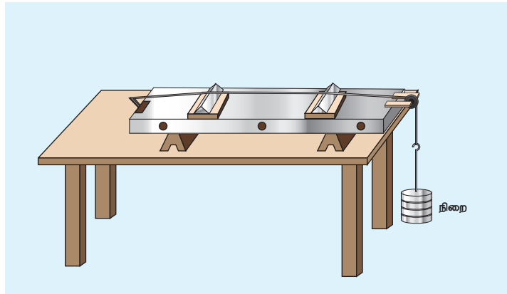
படம் 11.34 சுரமானியின் (sonometer) தோற்றம்
