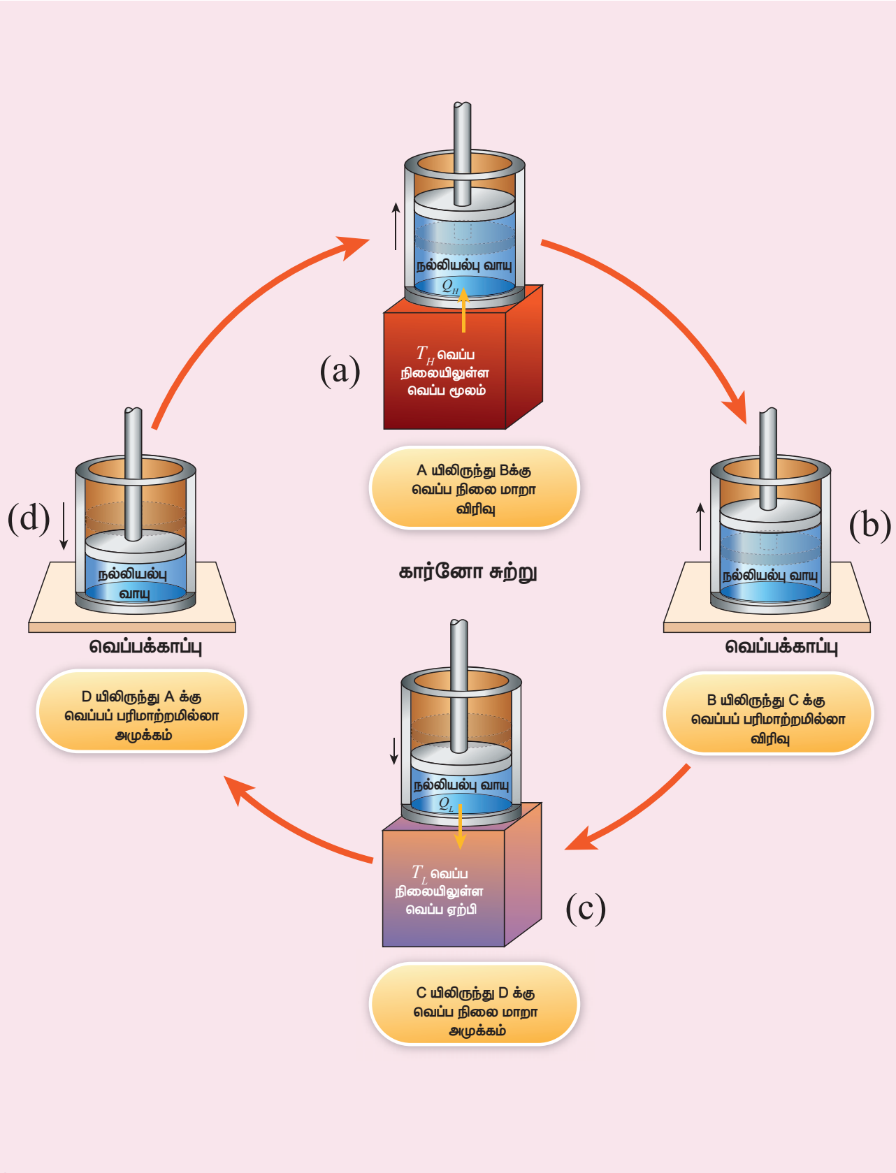
படம் 8.47 கார்ட்னோ சுற்று
