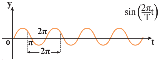
படம் 11.25 சைன் வடிவ சார்பு y = A \sin(\omega t) யின் வரைபடம்
