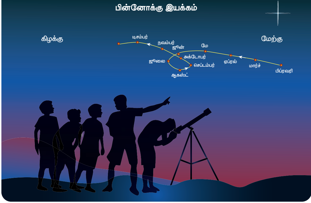
படம் 6.25 பின்னோக்கிச் செல்வதுபோல் தோன்றும் இயக்கம்
