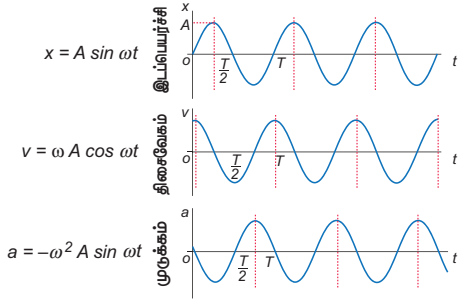
படம் 10.10 வெவ்வேறு கணநேரத்தில் இடப்பெயர்ச்சி, திசைவேகம், முருக்கத்தின் மாறுபாடு
