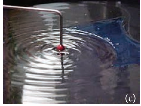
படம் 11.2 (a) கடலில் தோன்றும் அலைகள் (b) ரப்பர் பேண்ட் இழுத்துவிடப்பட்டதால் நிலை அலைகள் மற்றும் (c) நீர்ப்பரப்பில் உருவான சிற்றலைகள்
