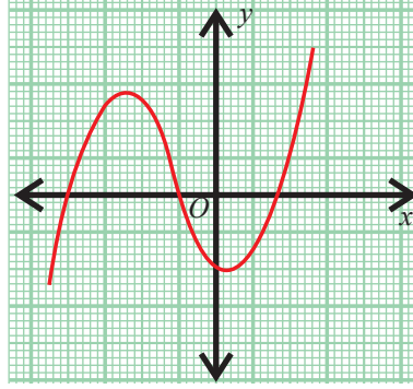
y = (x+4)(x+1)(x-2) , மூப்படி பல்லுறுப்புக்கோவை
