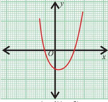
y = (x+1)(x-2) , இருபடி பல்லுறுப்புக்கோவை
