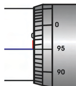
எதிர்ப் பிழை
