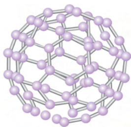
படம் 13.8 ஃபுல்லரீன்
