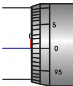
சுழிப் பிழை
