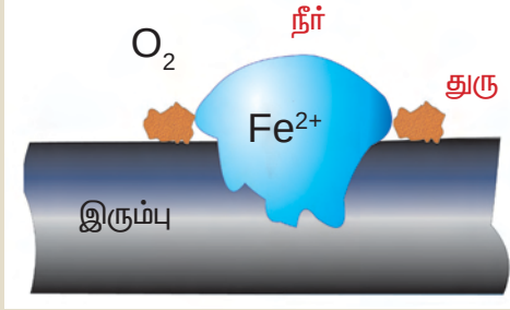
இரும்பு துருப்பிடித்தல்
