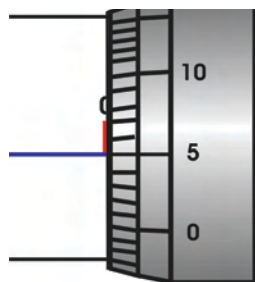
நேர்ப் பிழை
